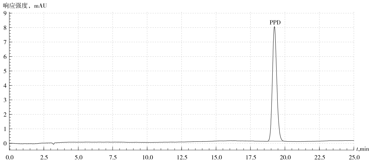
图 A.1 100 mg/L 苯基磷酸二胺标准品液相色谱图
