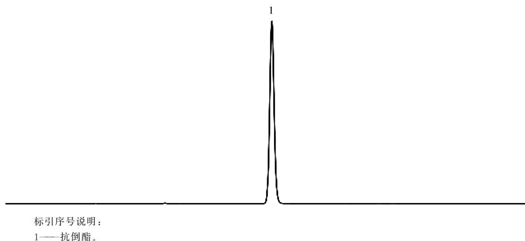
图 2 抗倒酯原药的高效液相色谱图
