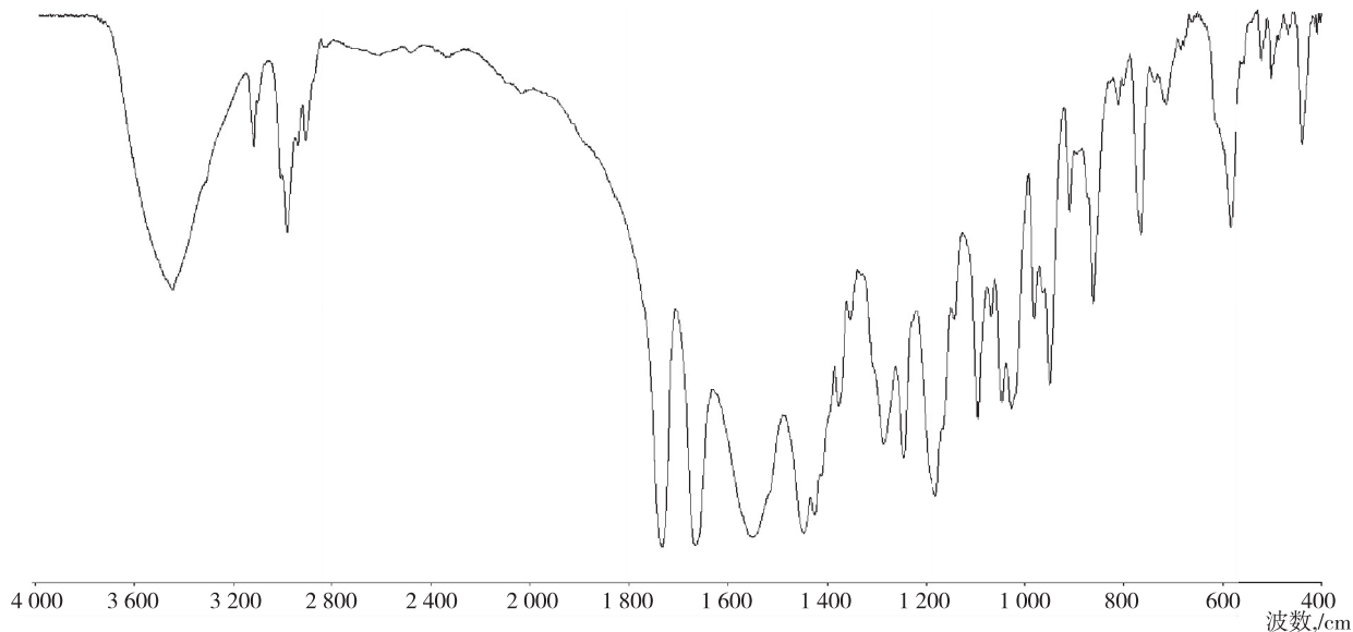
图 1 抗倒酯标样的红外光谱图
