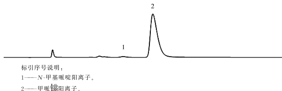
图 2 甲哌鎓可溶液剂阳离子色谱图
