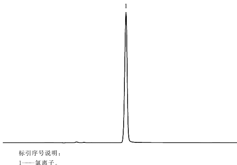
图 1 甲哌镱可溶液剂离子色谱图(测定氯离子)
