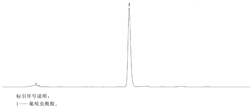
图 1 氟啶虫酰胺水分散粒剂的高效液相色谱图
