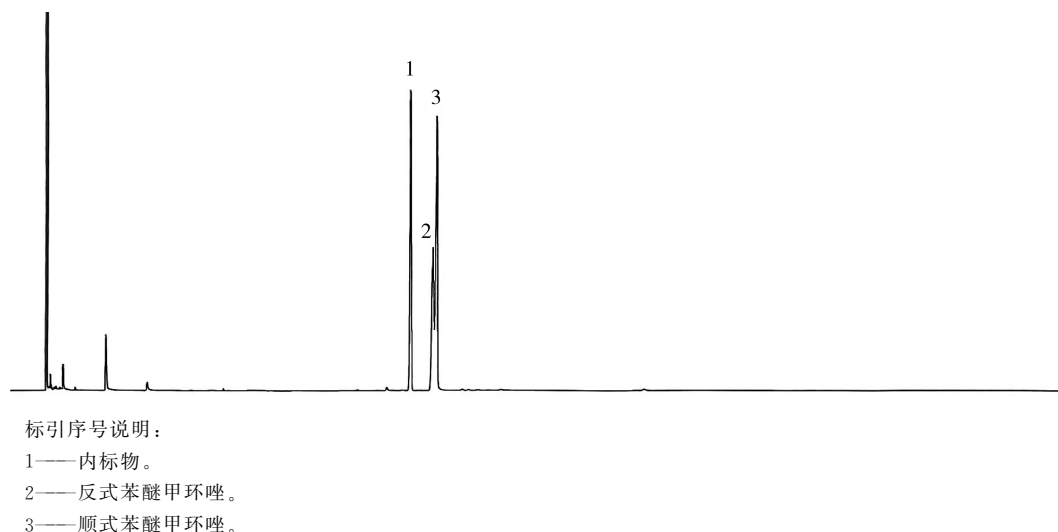
图 1 苯醚甲环唑水分散粒剂与内标物的气相色谱图
